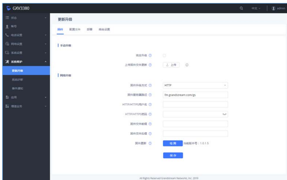
图 10: GXV3380 通过 Web UI 升级
